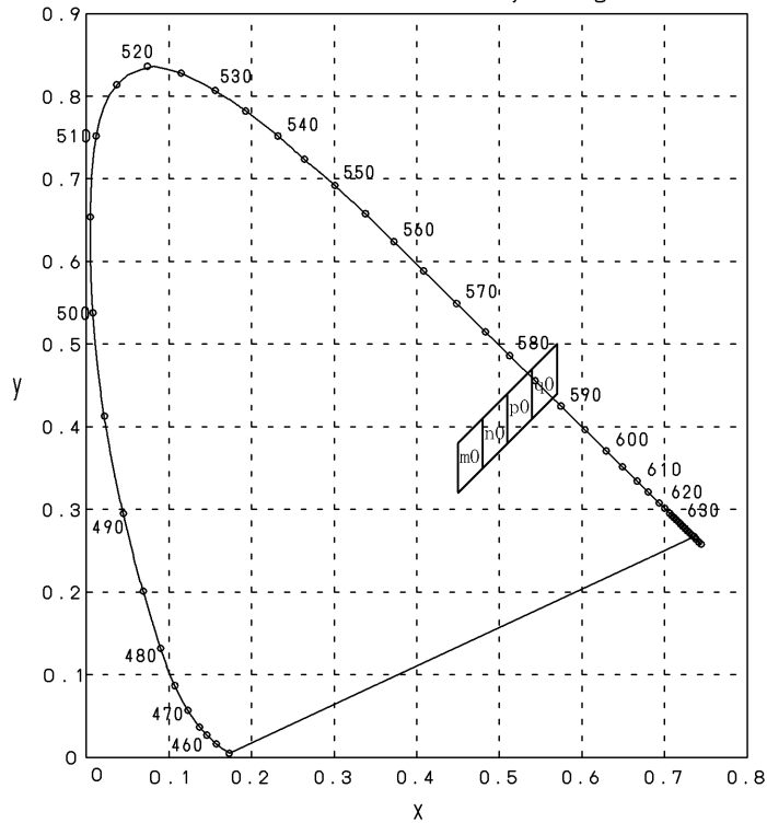
色度図 / Chromaticity Diagram
